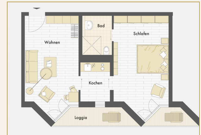
Beispielgrundriss einer 2-Zimmer-Wohnung – weitere Wohnungsgrößen und Grundrissvarianten stehen zur Auswahl.
